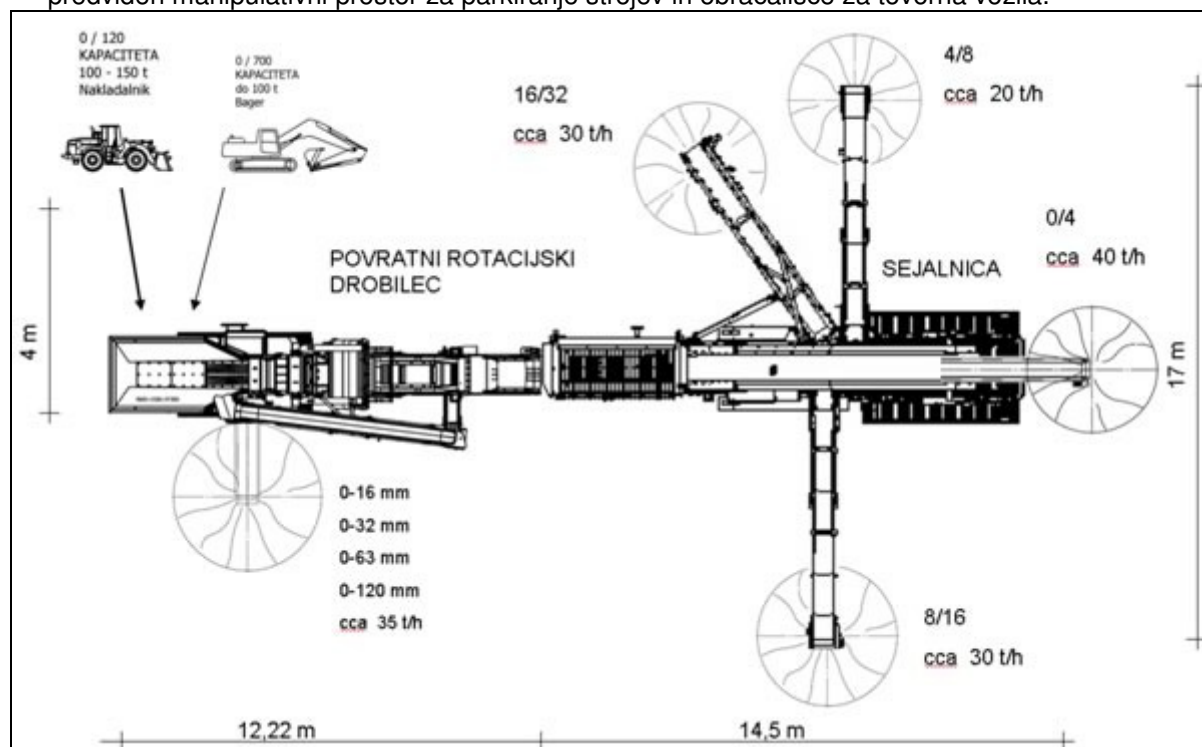
Shematski prikaz tehnološke opreme na osnovni etaži
