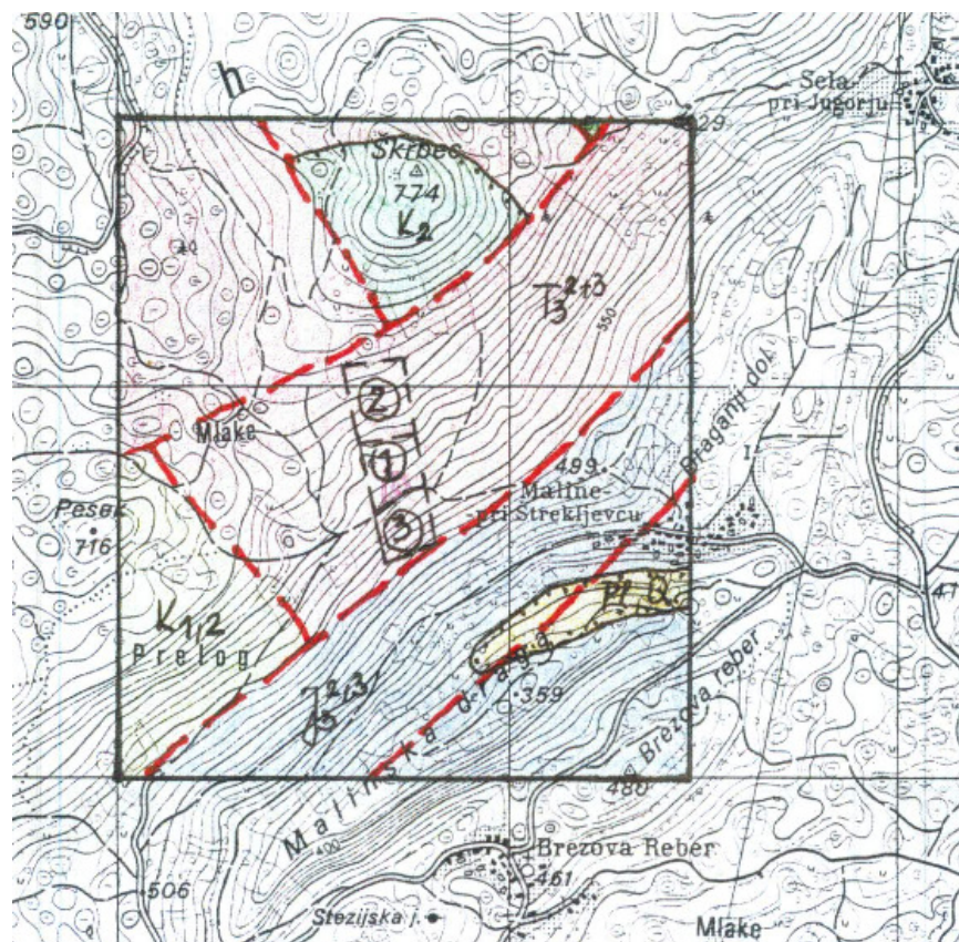
Slika 1: geološka situacija
