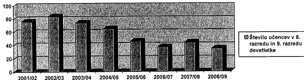
Graf 2: Število otrok, ki so obiskovali v zadnjih osmih letih 8. razred oz. 9. razred devetletke
